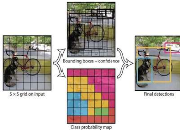
Fig. 5 - The Yolo process [18]
