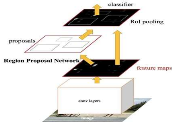
Fig. 6 - Faster_ R-CNN step [18]
